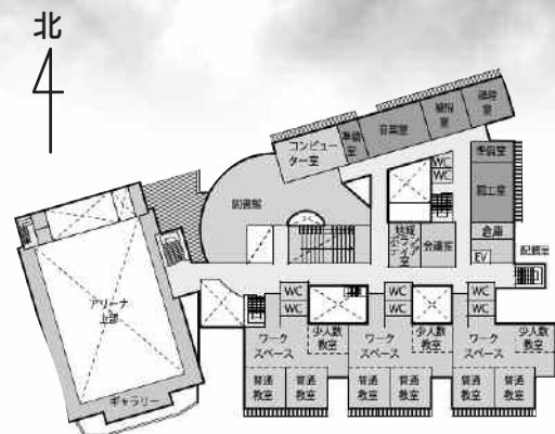
▲2階平面図
