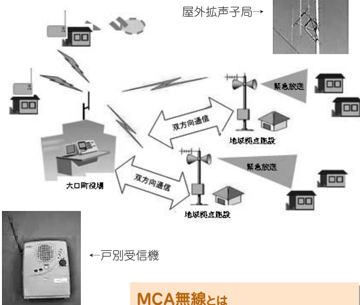
■デジタル防災行政無線のイメージ図
