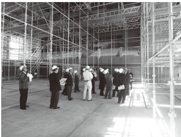
中央公民館集會室の耐震工事の様子
