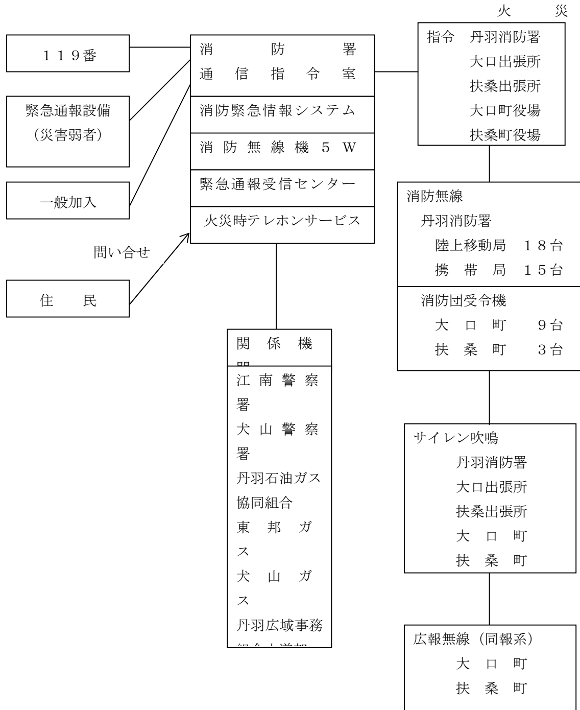
S2-24 丹羽広域事務組合消防本部通信系統図
